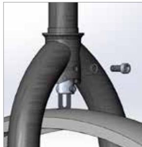
図2：フェンダーフルートをステアリングコラムに取り付けます。
